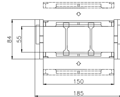
SECTION A-A (S=2:1)
